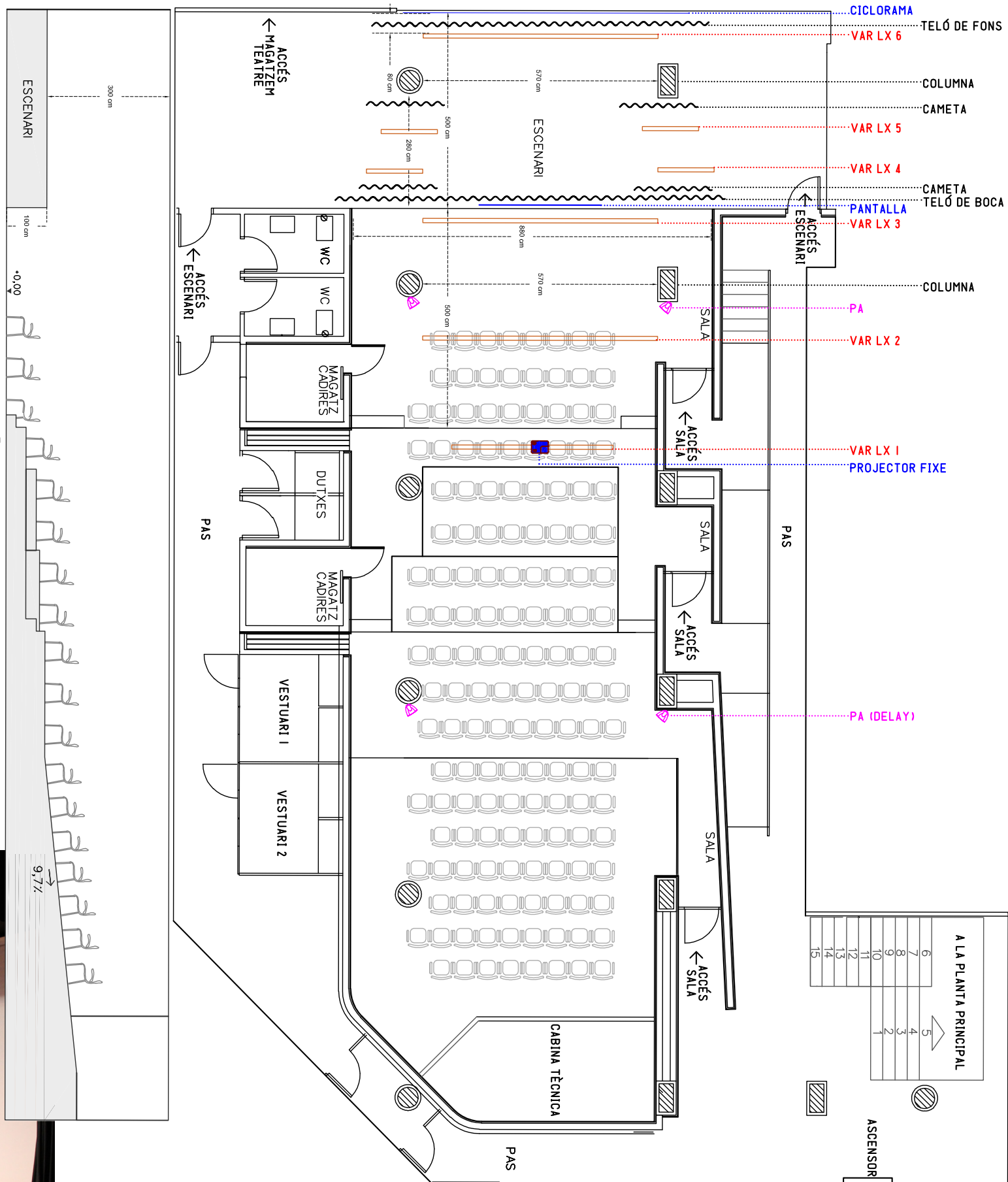
PLANOL: SALA TÍSNER - DISPOSICIÓ D'ELEMENTS VERSIO: 1.0
